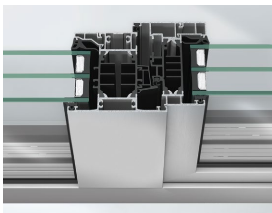
Schüco AW CT 72 combinación de luz fija y hoja
