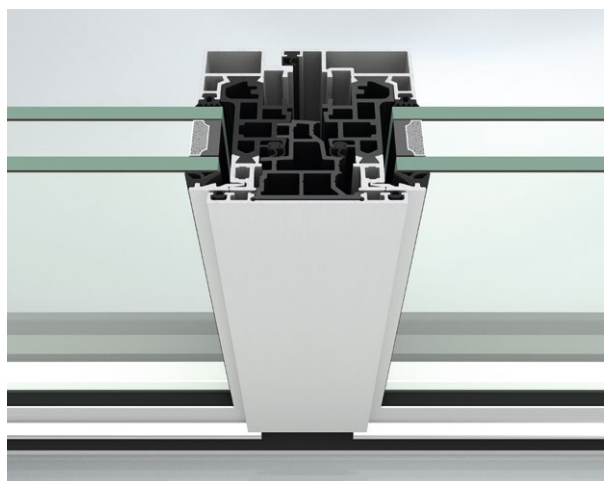
Schüco AW CT 72 BS doble hoja
